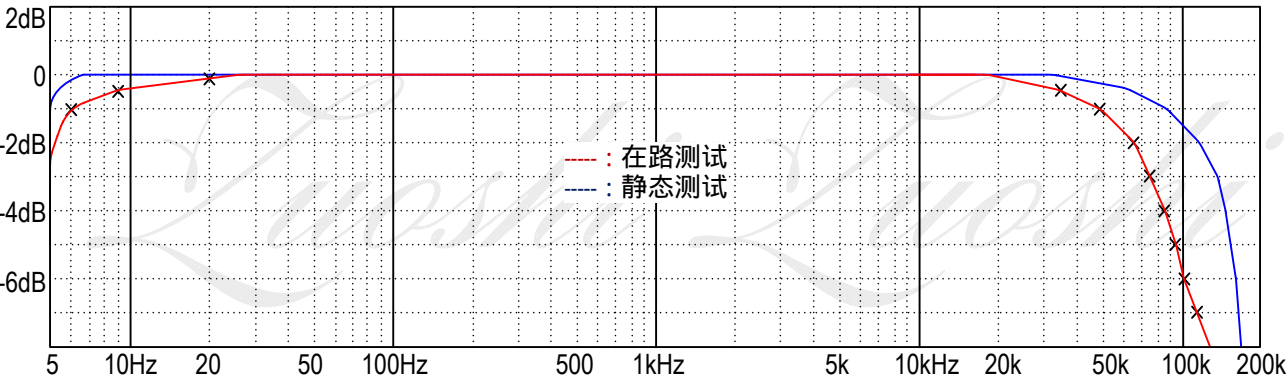
图3. 频响曲线
